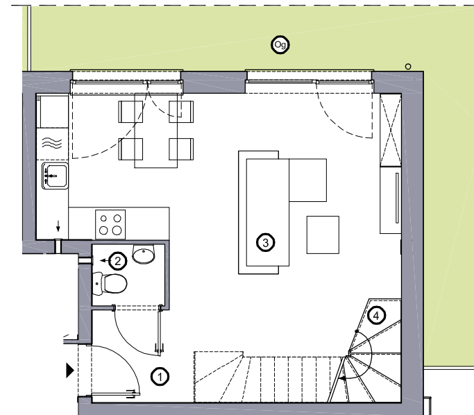
Rzut parteru
