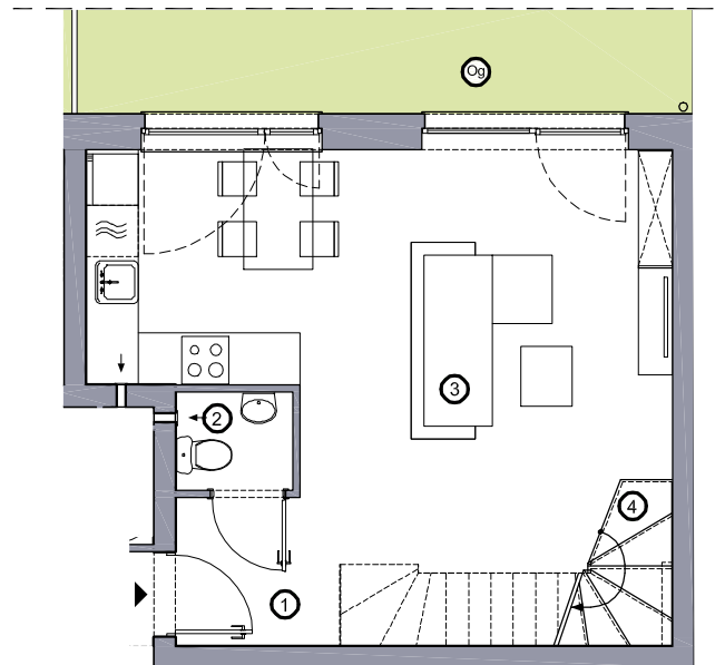
Rzut parteru
